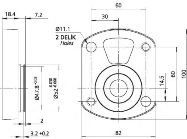
D KAPAK TİPİ / Flange type
