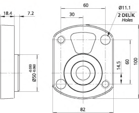
F KAPAK TİPİ / Flange type
